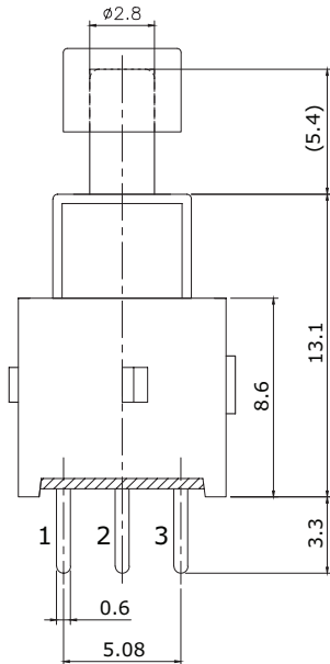
5.4 MM ACTUATOR
