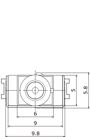
5.4 MM ACTUATOR
