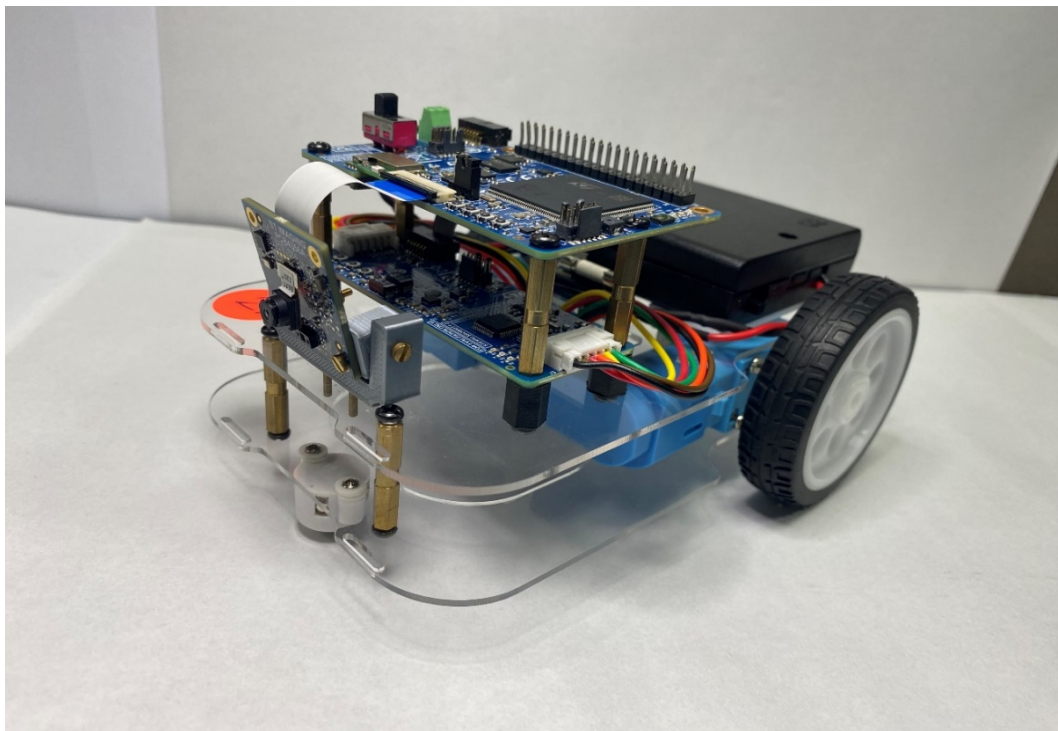
Figure 1. STEVAL-ROBKIT1
